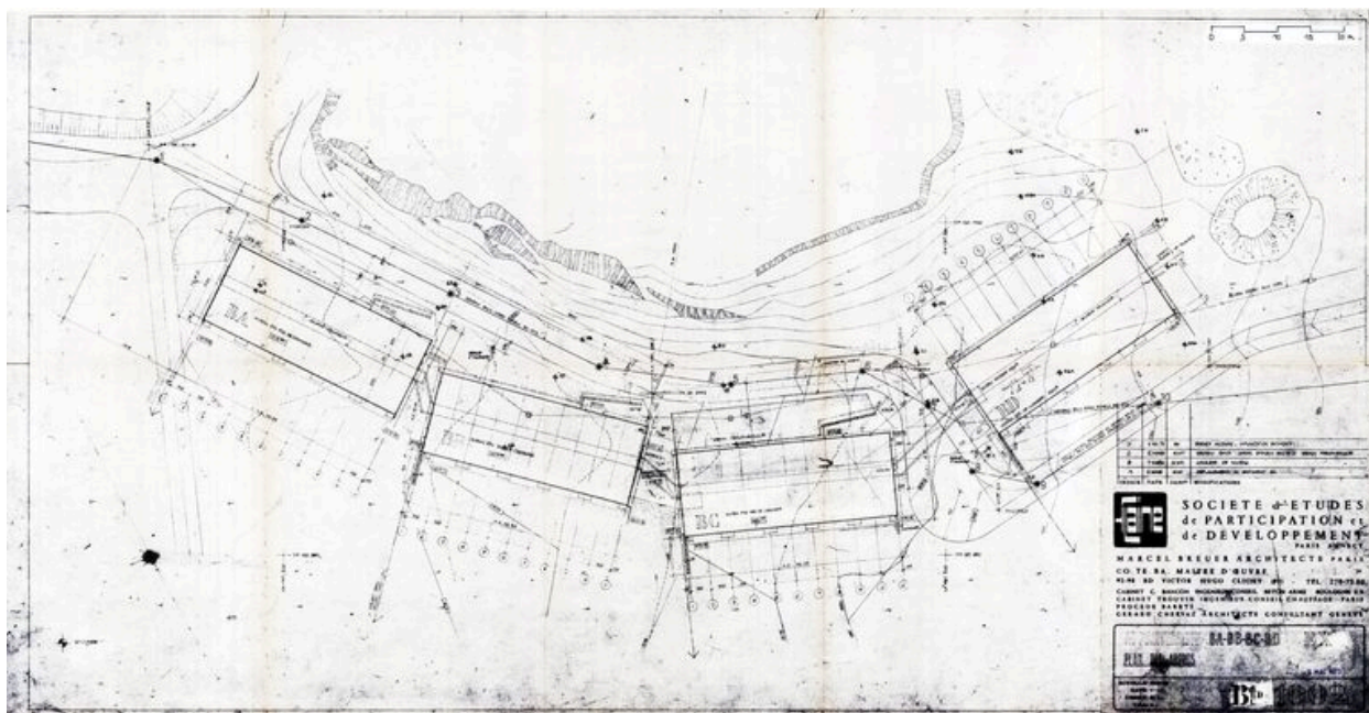
Plan des abords. Marcel Breuer architecte, 27 novembre 1972 (AC Magland)
