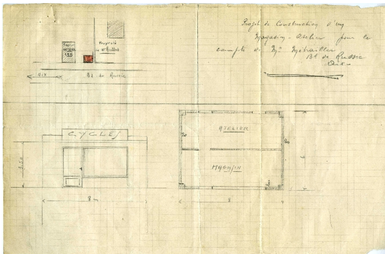
Projet de construction d'un magasin et atelier, 1934
