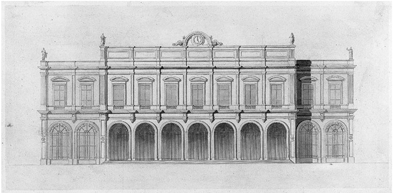
Projet de gare, non réalisé, par l'architecte Henri Feuga : élévation principale du bâtiment-voyageurs
