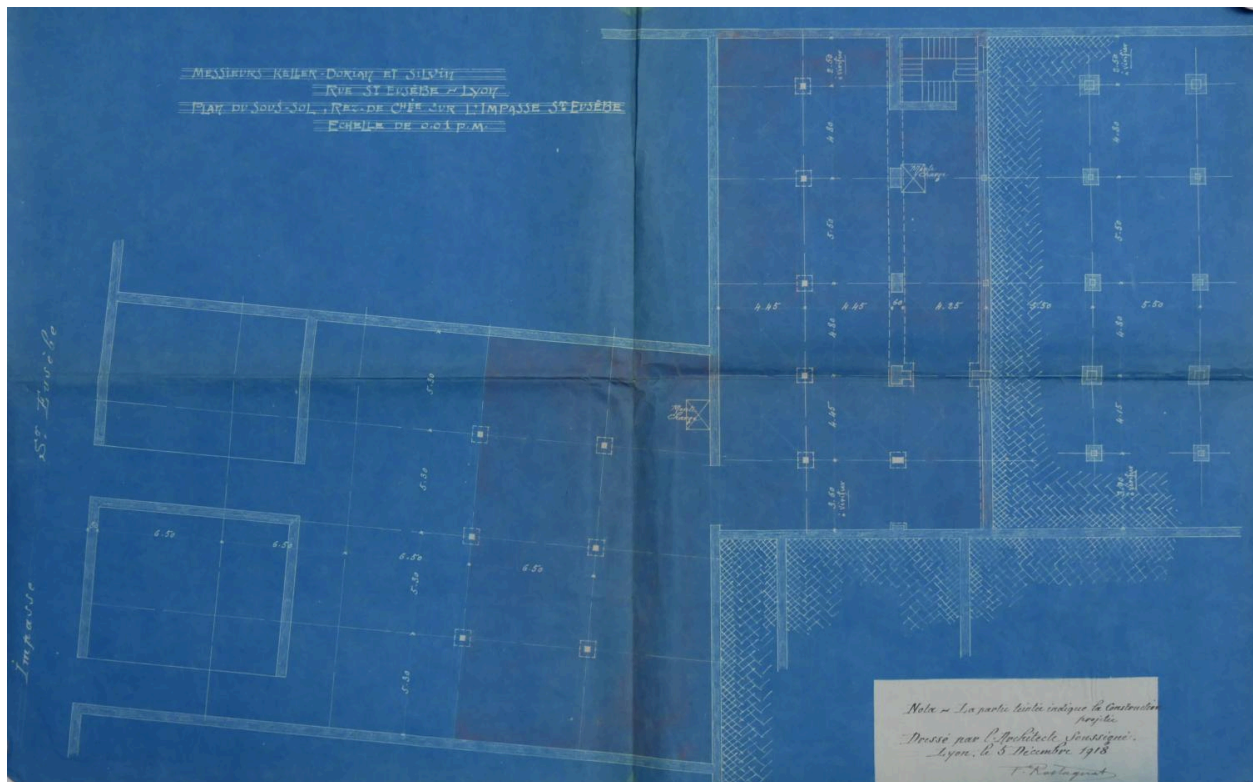
Plan du rez-de-chaussée sur la rue St-Eusèbe 1918 (AC Lyon 314W/595)
