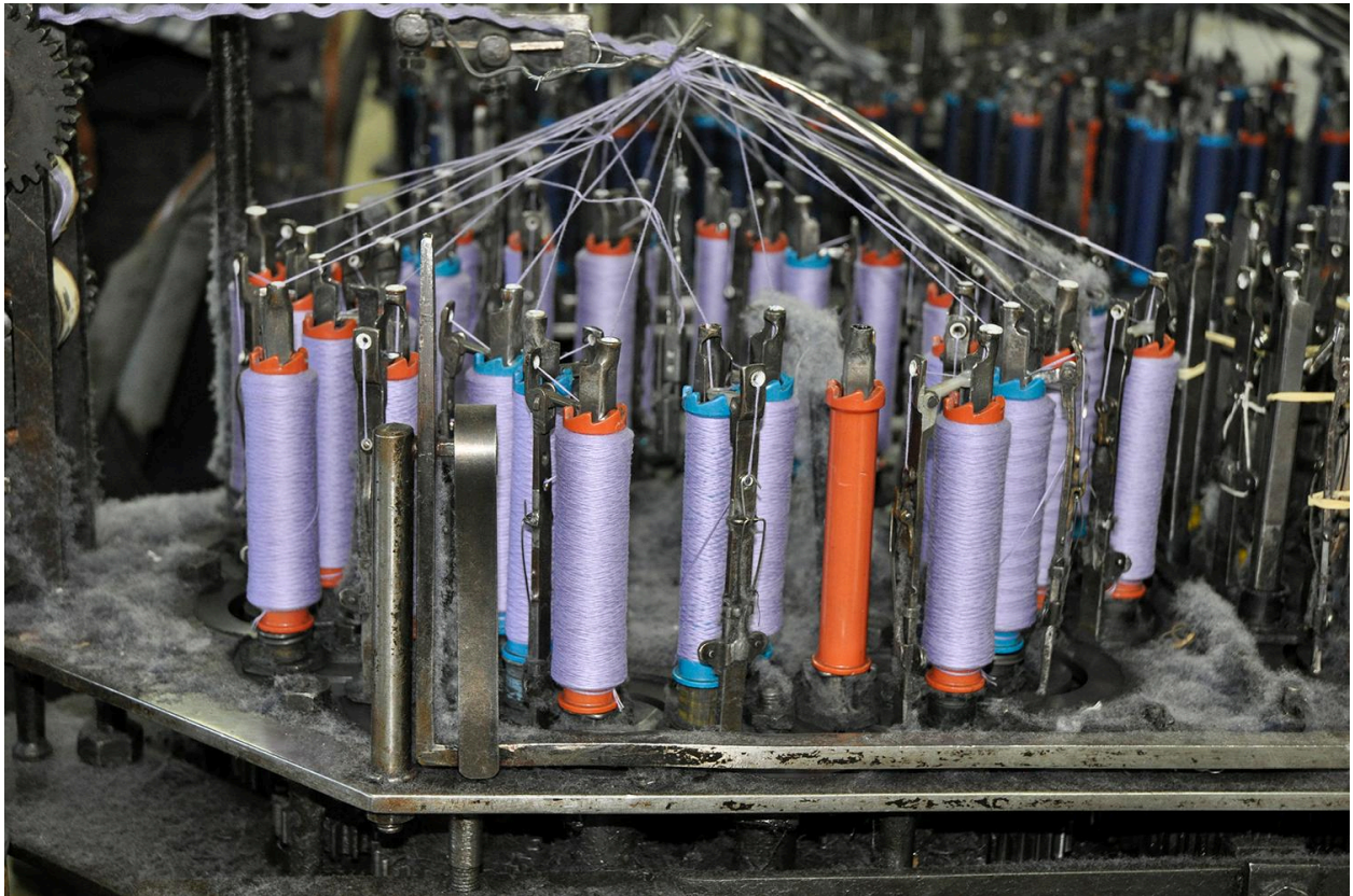
Détail bobines du métier des tresses
