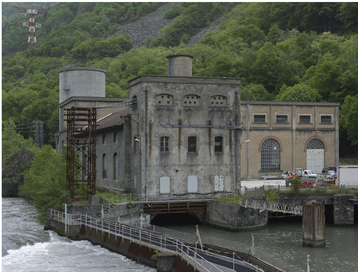
Vue d'ensemble de la centrale
