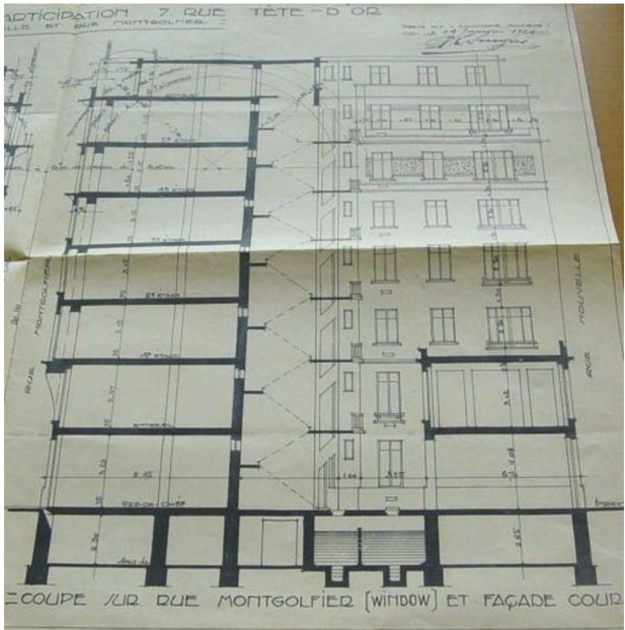
Coupe sur rue Montgolfier et façade sur cour
