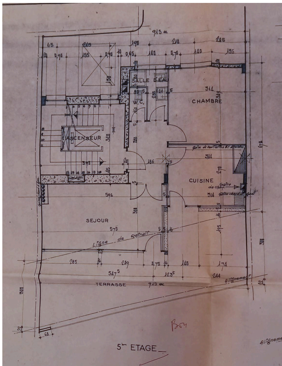
Plan du cinquième étage, 29 avenue d'Italie
