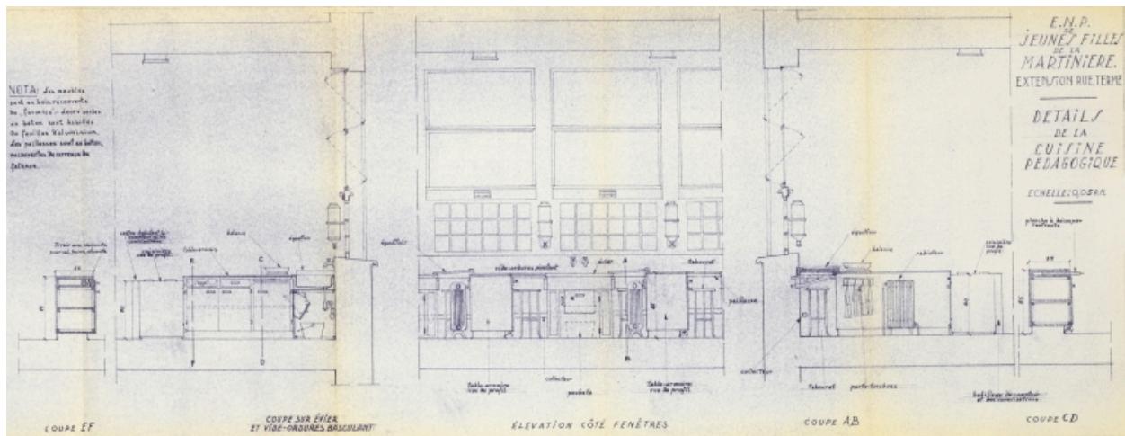
Détails de la cuisine pédagogique. 1:50. Document figuré. Coupe. Archives du Lycée de la Martinière (intendance Augustins). non coté
