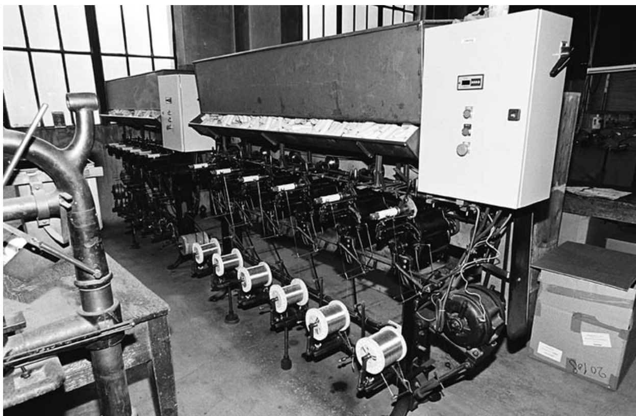
Machine à bobiner et à guiper vue d'ensemble
