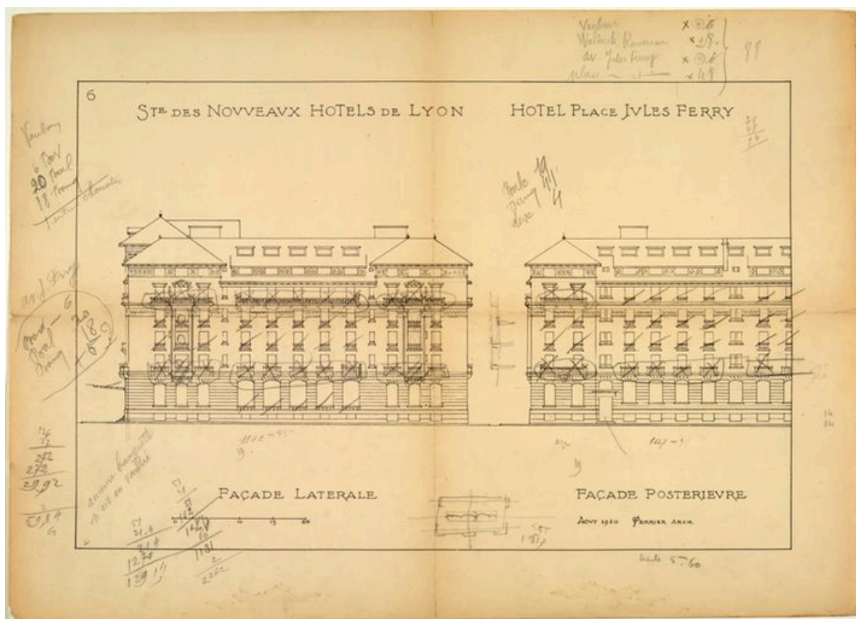
Elévations latérale et postérieure, Valère Perrier architecte, 1920
