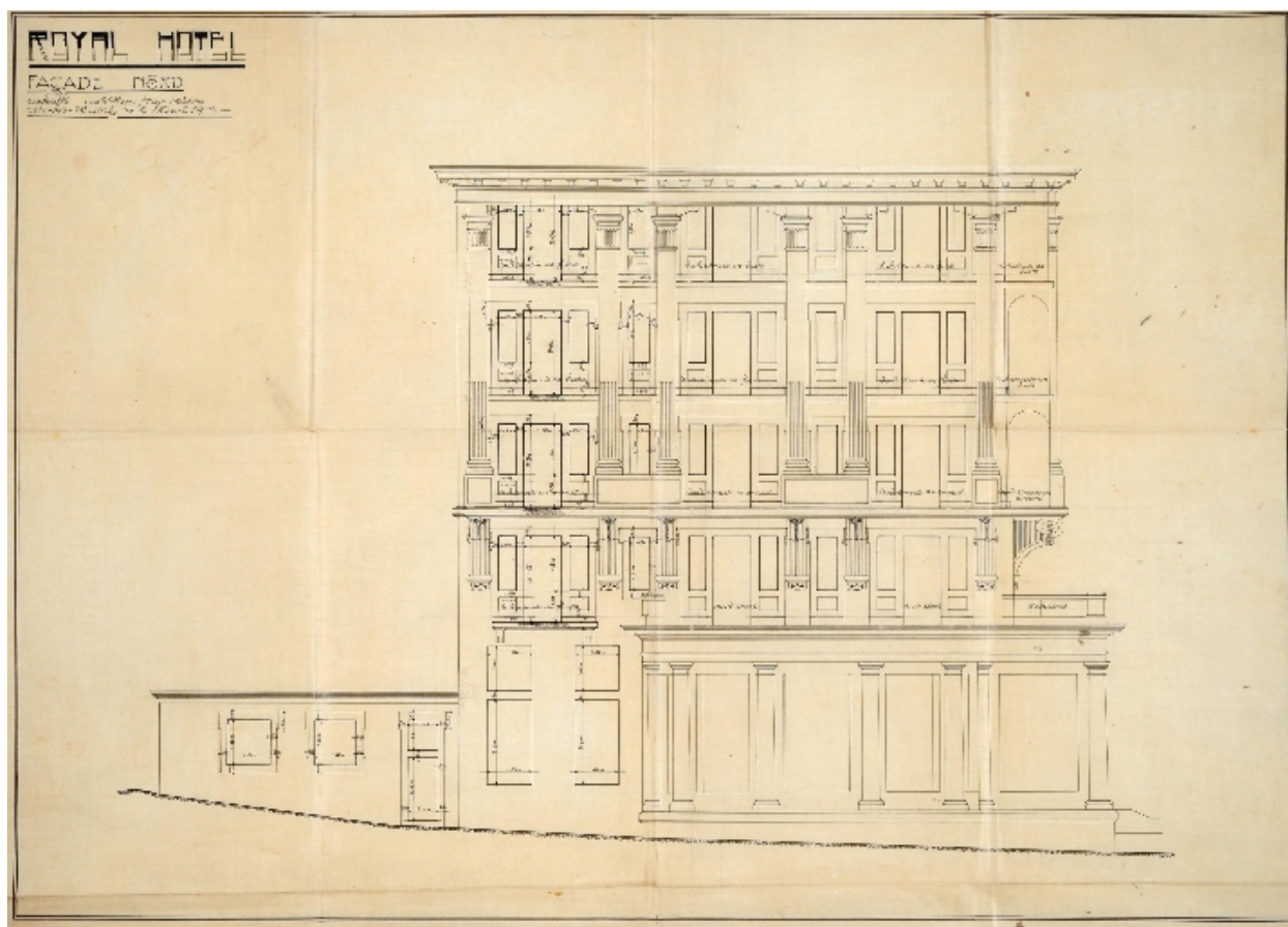
Elévation nord, 1914
