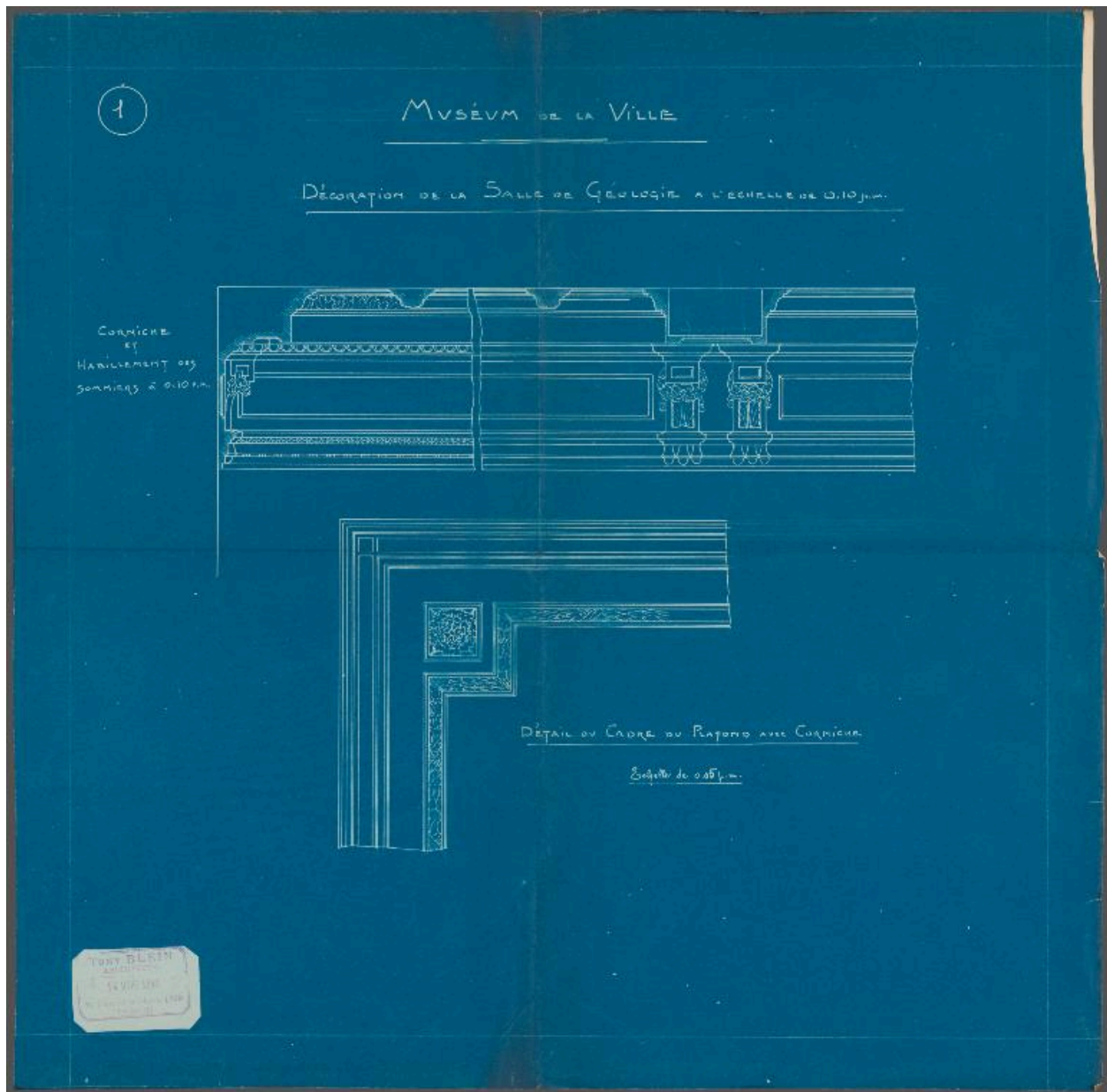
Décoration de la salle de Géologie, corniche et habillage des sommiers, détail du cadre du plafond avec corniche, Tony Blein architecte, 14 mars 1913. AC Lyon, 515 Wp 6 2
