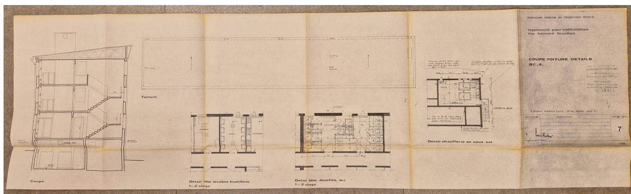
Coupe transversale, toiture et détails du bâtiment A de la rue Bernard-Brunhes, par Daniel Michelin, 1967.
