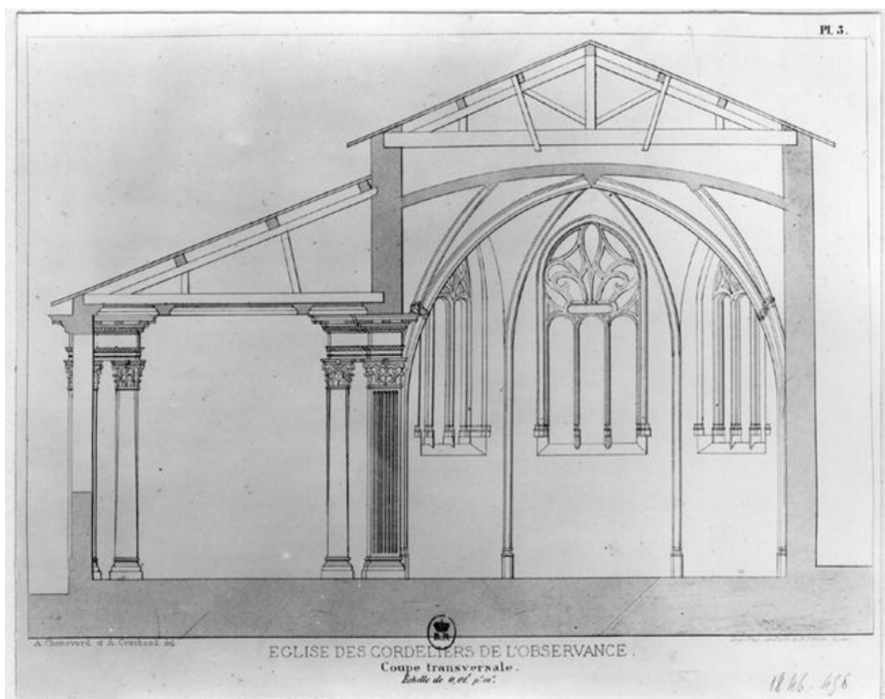
Eglise des Cordeliers de l'Observance. Coupe transversale
