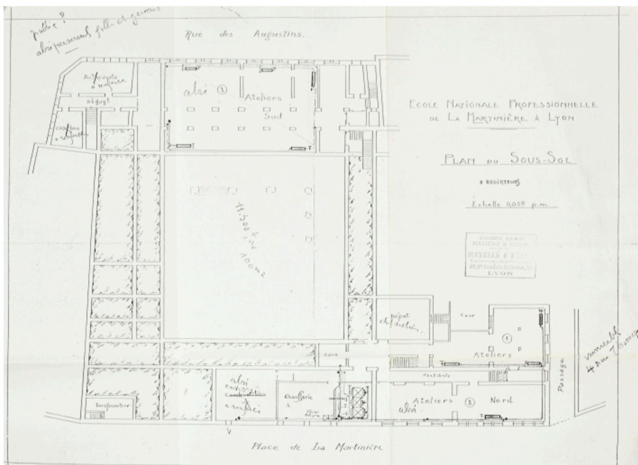
La Martinière 9 rue des Augustins Lyon. Plan du sous-sol. Ech. 0,01 m par mètre. Document figuré. Sans date. 1:100. Archives du Lycée de la Martinière (intendance Augustins). non coté
