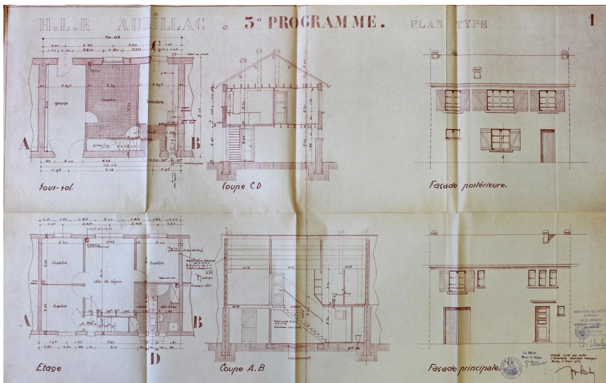
Aurillac, cité des Camisières, plans, coupes et élévations d'une maison HLR du 3e programme, dessin daté par erreur de mars 1953, vraisemblablement créé en mars 1954, Jacques Porcher architecte (Archives départementales du Cantal, 36 W 19, chemise « Camisières 3e programme »)
