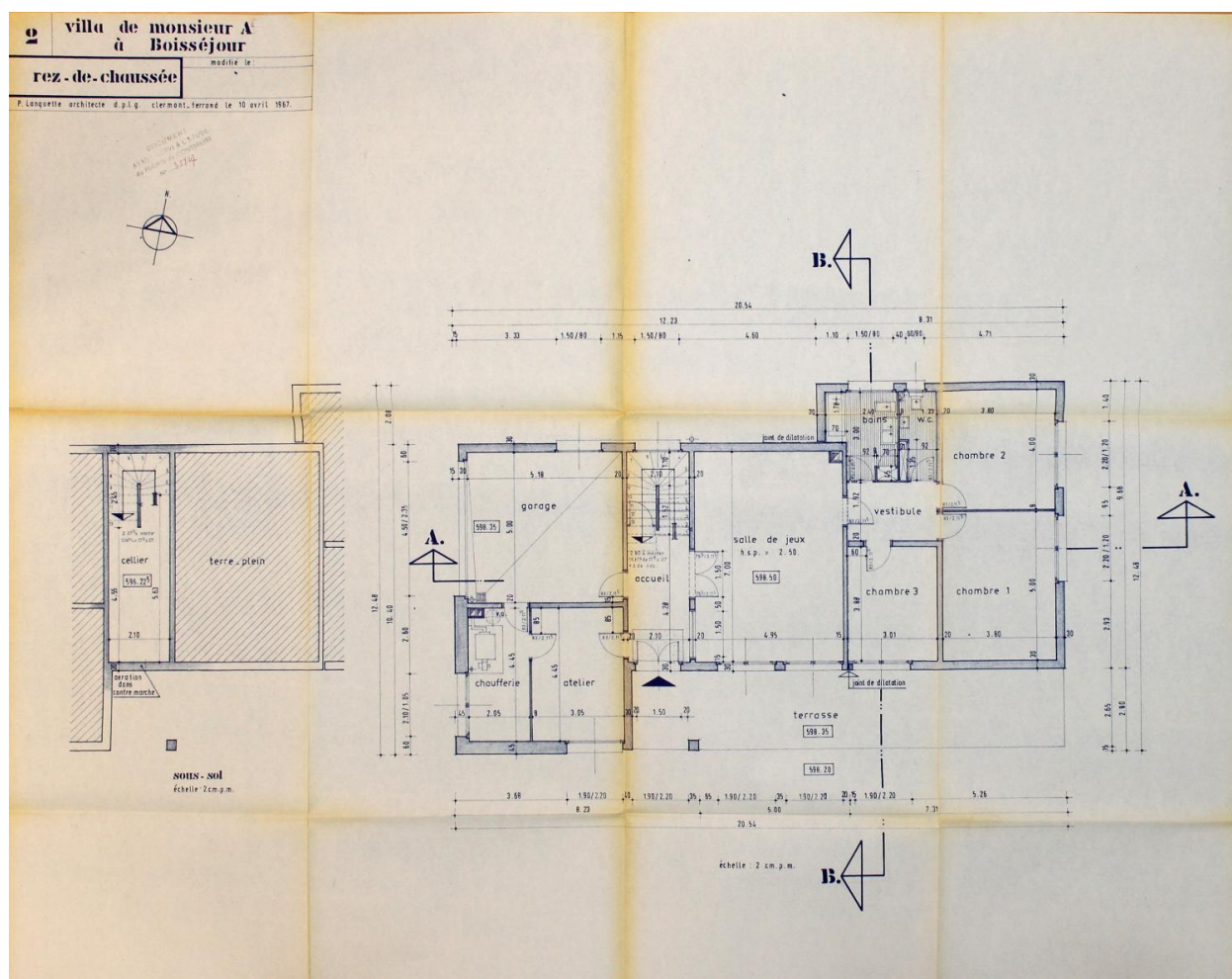
Ceyrat, la maison A., plan du rez-de-chaussée, Paul Lanquette architecte, avril 1967 (archives départementales du Puy-de-Dôme).
