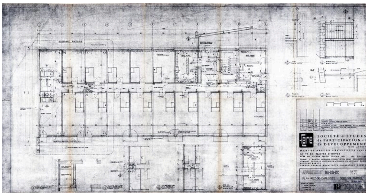
Plan du rez-de-chaussée et du sous-sol partiel. Marcel Breuer architecte, 27 novembre 1972 (AC Magland)
