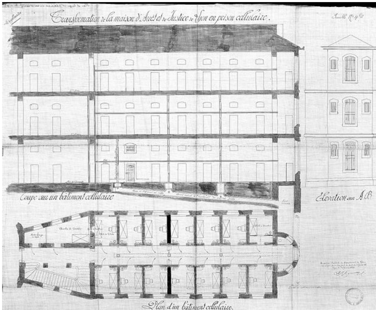
Transformation de la maison d'arrêt et de justice de Lyon en prison cellulaire : plan et coupe d'un bâtiment cellulaire, élévation sur A-B, H. Moncorger, 1885. calque entoilé, 10 janvier 1885, 69 x 83,5 AD, Rhône. 1 Y 283
