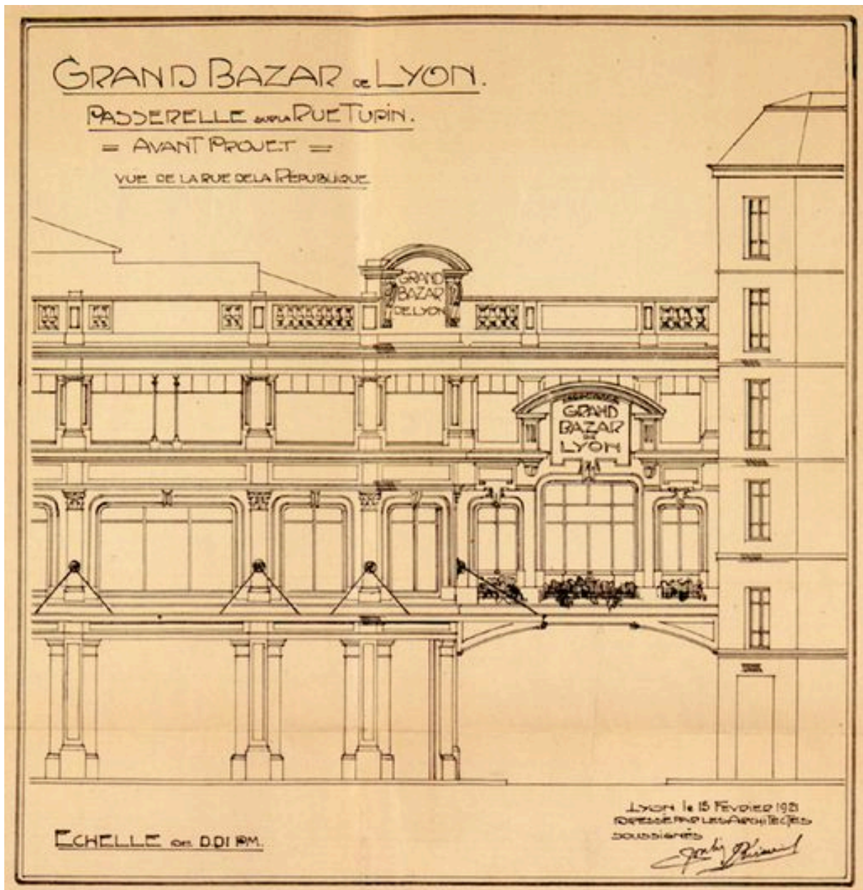
Grand Bazar de Lyon. Passerelle sur la rue Tupin. Avant-Projet. Vue de la rue de la République / J. Bissuel, H. Joulie, 15 février 1921 (Arch. mun. Lyon. 922 WP 1097)
