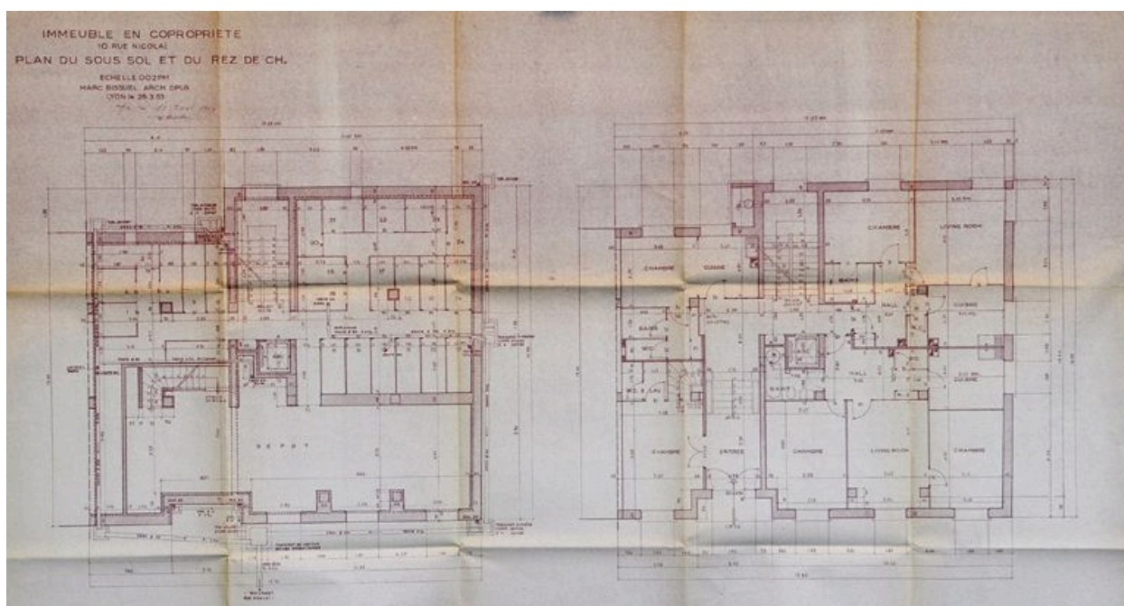
Plan du sous-sol et du rez-de-chaussée, par Marc Bissuel, 28 mars 1953 (AC Lyon, 1097 W 559)
