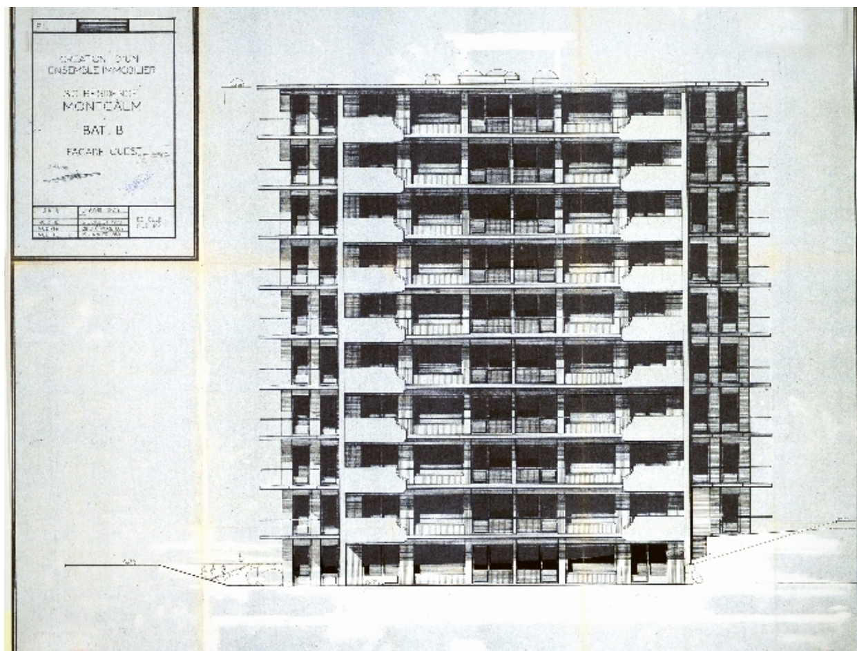
Bât. B : élévation ouest
