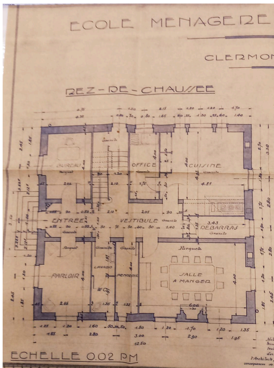
Ecole ménagère, internat : Plan du rez-de-chaussée
