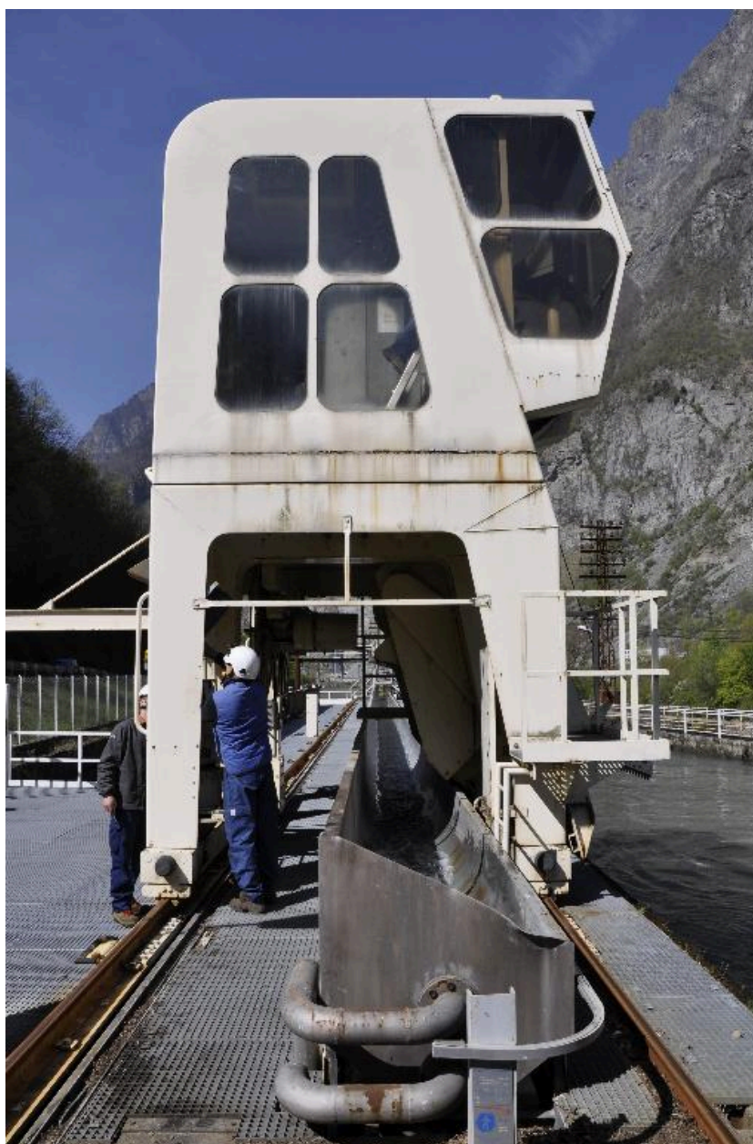
Vue du dégrilleur cabine du barrage de Rioupéroux
