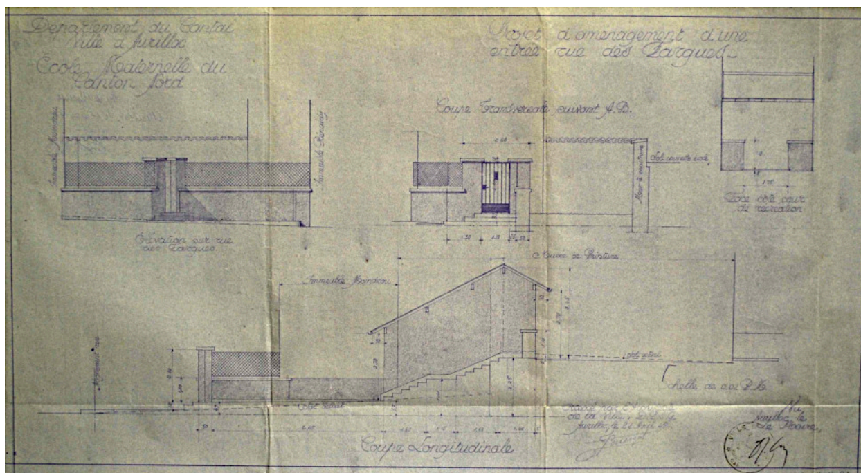
Projet d'aménagement de l'entrée rue des Fargues : coupes et élévations par J. Brunot, 1945 (AD Cantal, 2 O 14/14-21)
