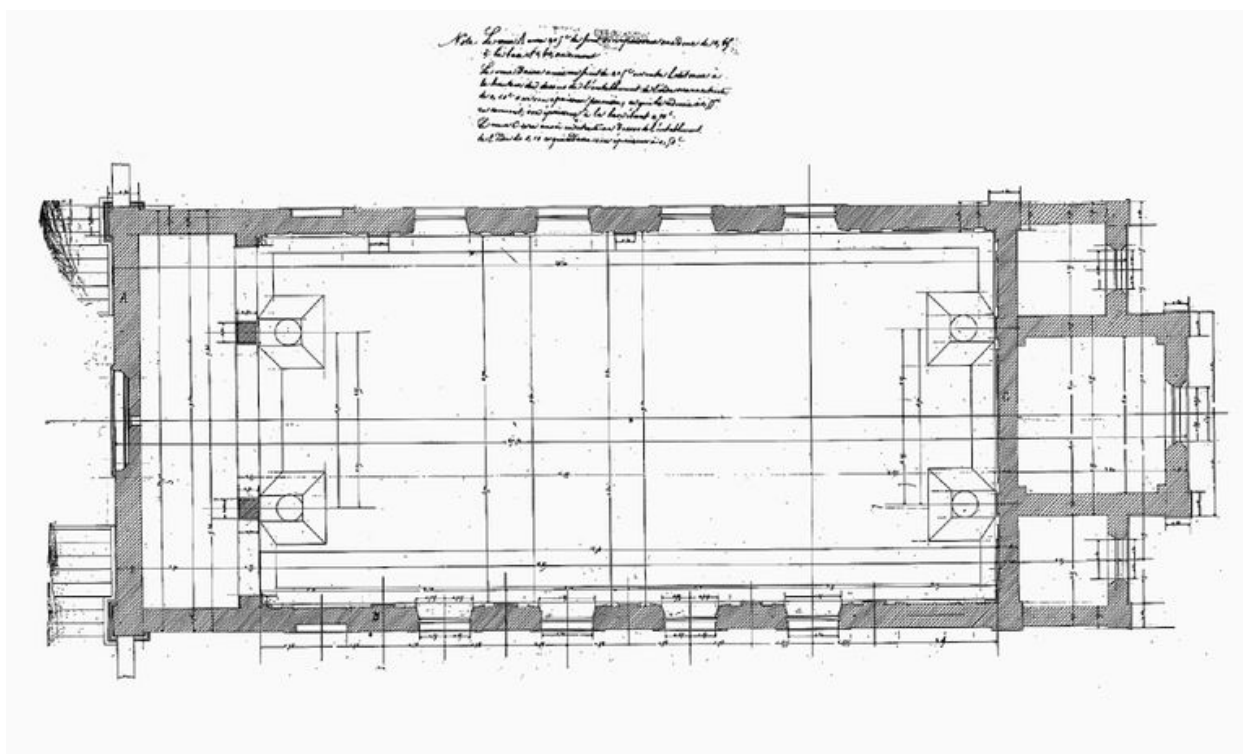
Chapelle de l'Observance, projet de plan
