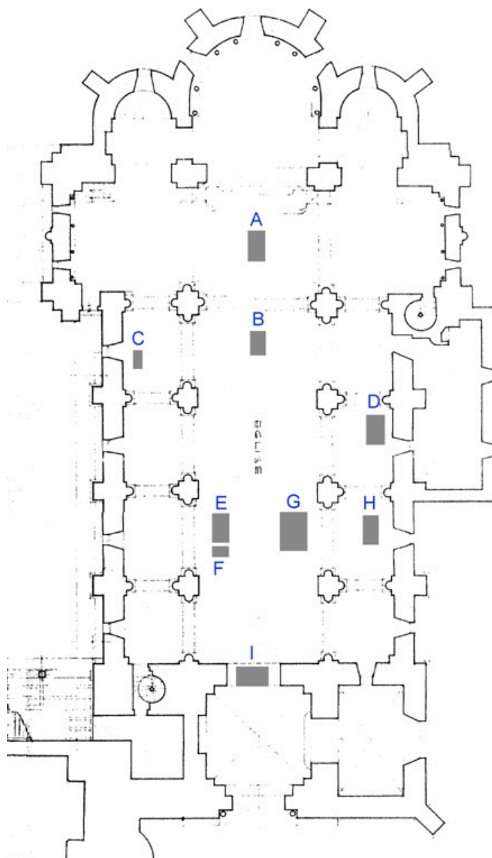
Plan de localisation des dalles funéraires (lettre G).
