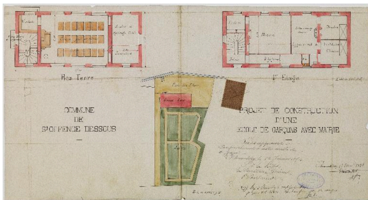
Projet de construction d'une école de garçons avec mairie, plans. Faga, 1893.
