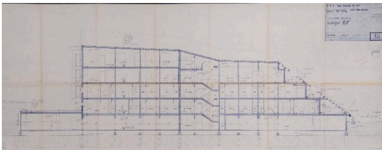
Les Cygnes, 1974 : coupe longitudinale
