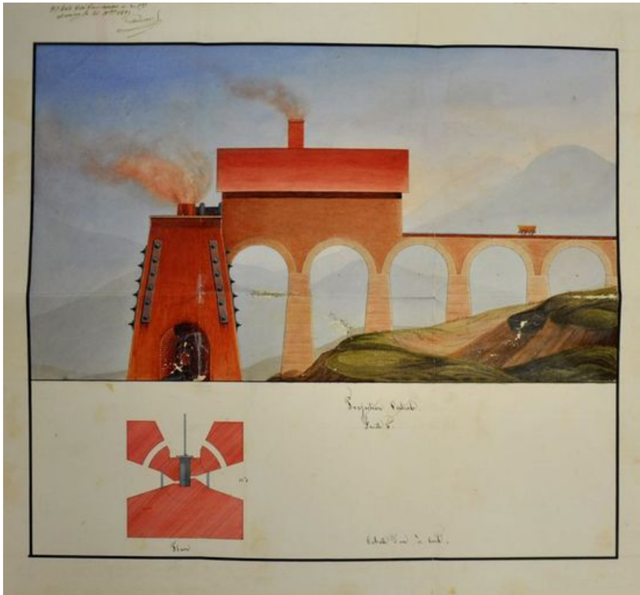
Elévation du haut fourneau. Plan. Archives départementales de la Haute-Savoie © Archives départementales de la Haute-Savoie. 10 FS 45
