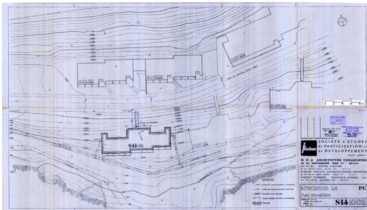
Plan des abords. M.B. A architectes urbanistes, 26 janvier 1984 (AC Arâches-la-Frasse)
