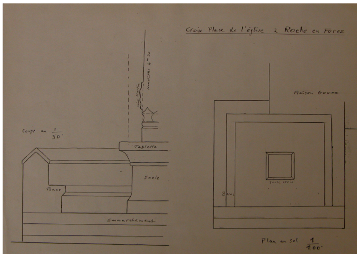
Croix place de l'église à Roche en Forez. Plan au sol 1/100°. Coupe au 1/50°. Dessin, 1972. AD Loire. 1111 VT 167
