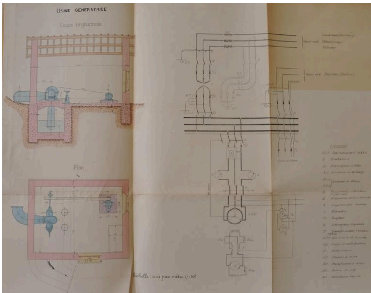
Plan accompagnant la demande de construction de la centrale, 1921 (FR.AD073, 83S28).
