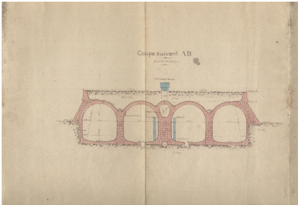
Coupe suivant AB
