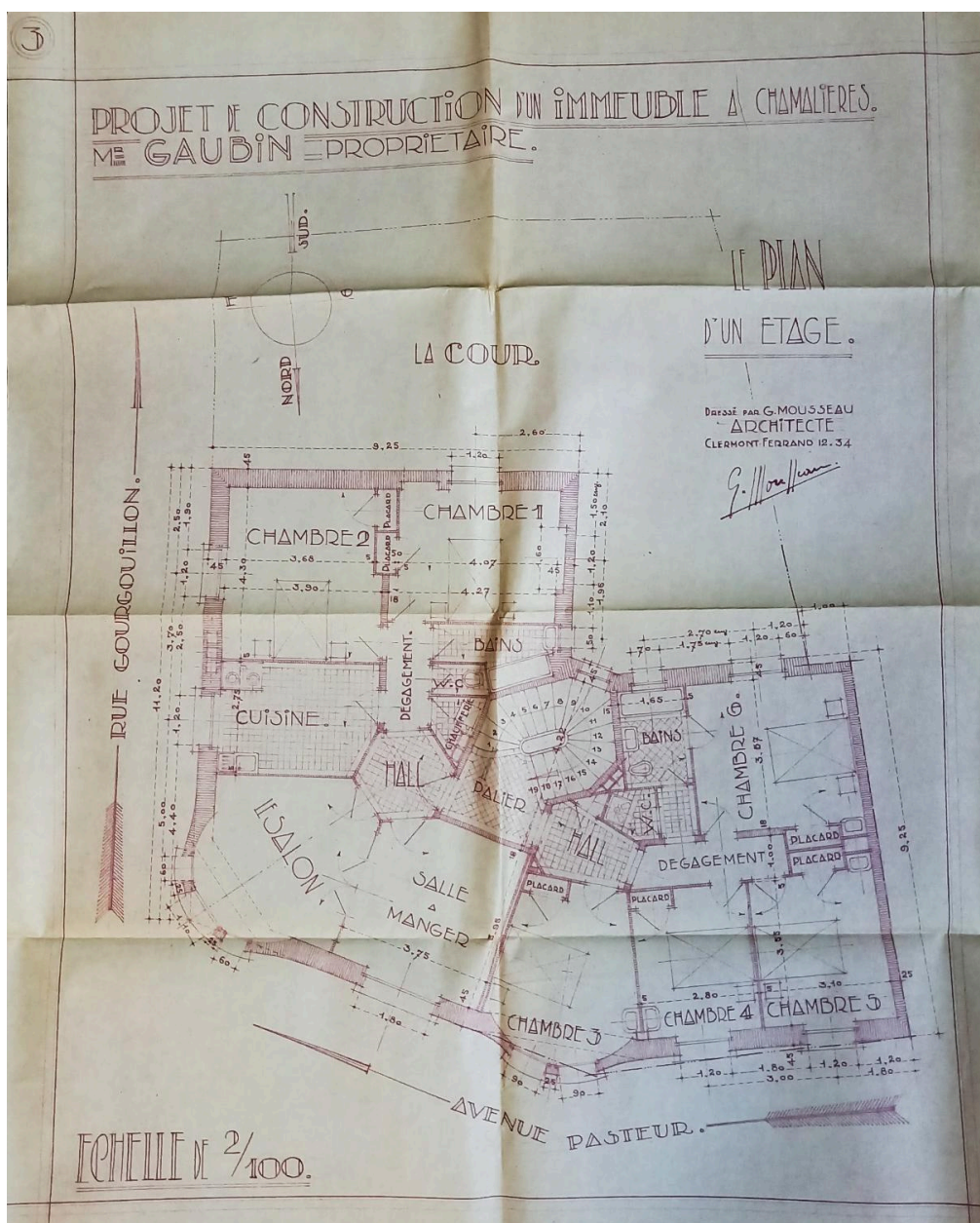
Plan d'un étage
