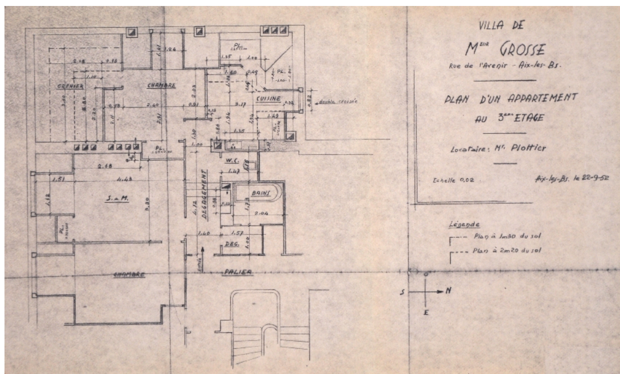
Plan de l'appartement du 3ème étage, 1952
