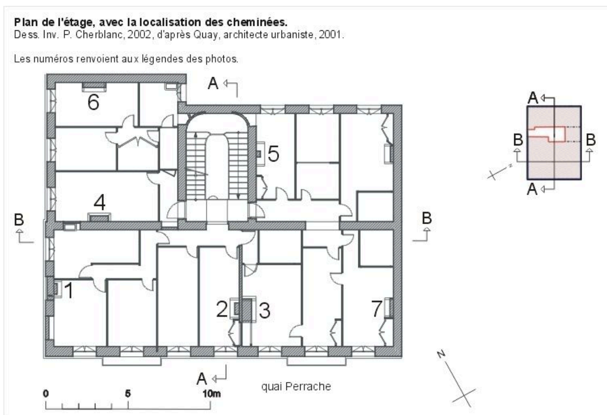
Plan du 1er étage avec localisation des cheminées
