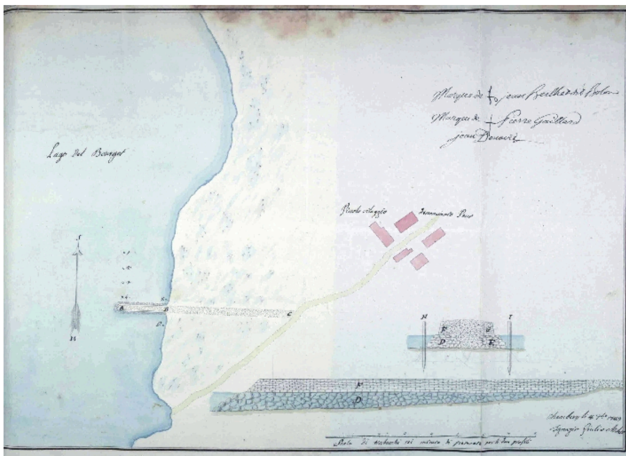
Plan et coupe du môle, 1783
