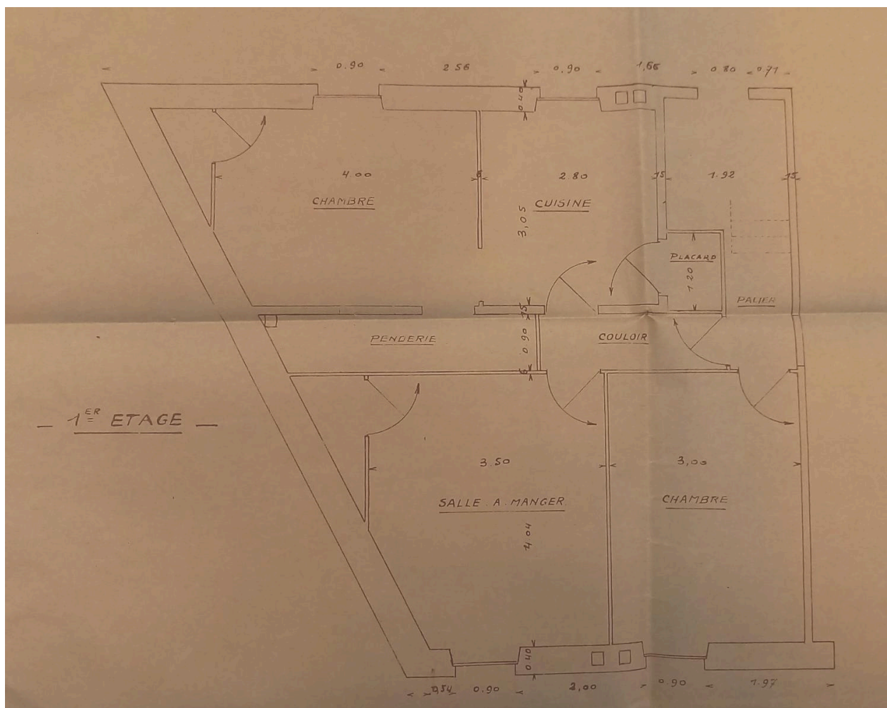
Plan de l'étage (comparaison)
