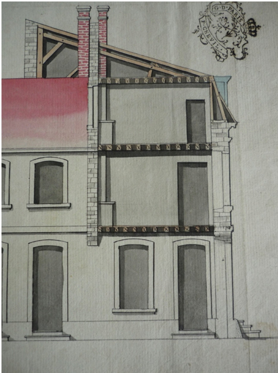
Elévation et coupe du corps de logis du grenier à sel, 17 mai 1740 (détail du côté droit). Plan AC Lyon. Fonds des HCL ; B421
