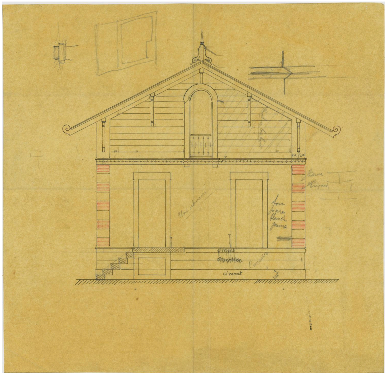
Villa Mireille : élévation est, [avant 1892]
