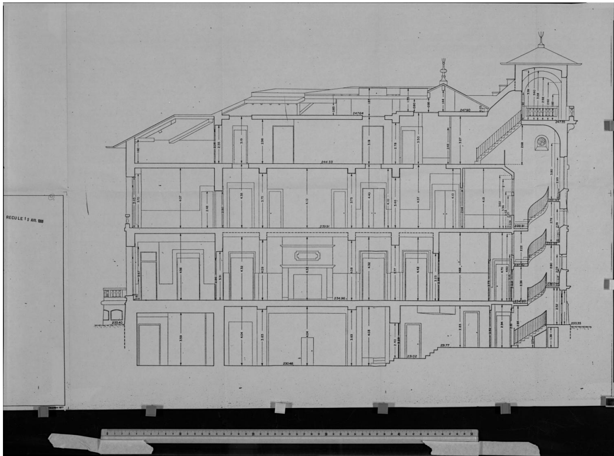
Coupe AA de la villa Gillet
