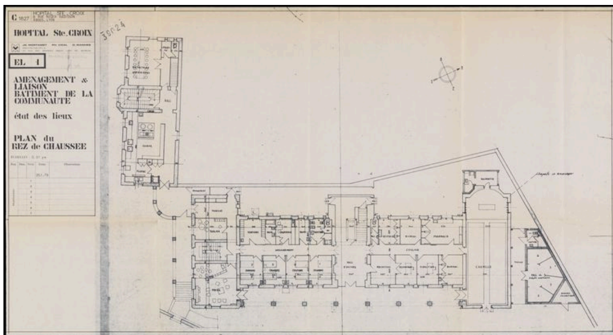
Plan du rez-de-chaussée, établi en 1979 (Arch. mun. Lyon, 905 WP_10, Agence Mortamet, Vidal, Manhes, tirage d'architecte).
