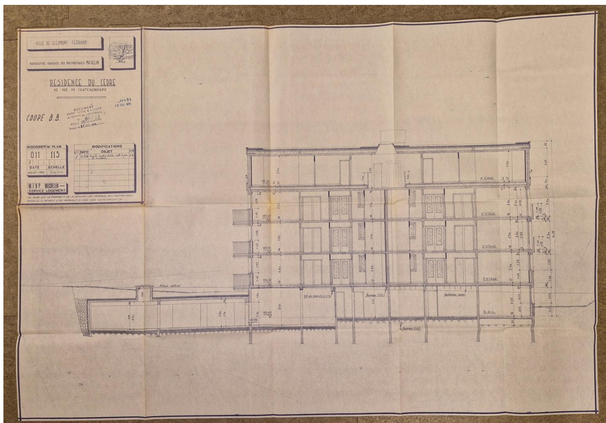
Coupe BB de l'immeuble.
