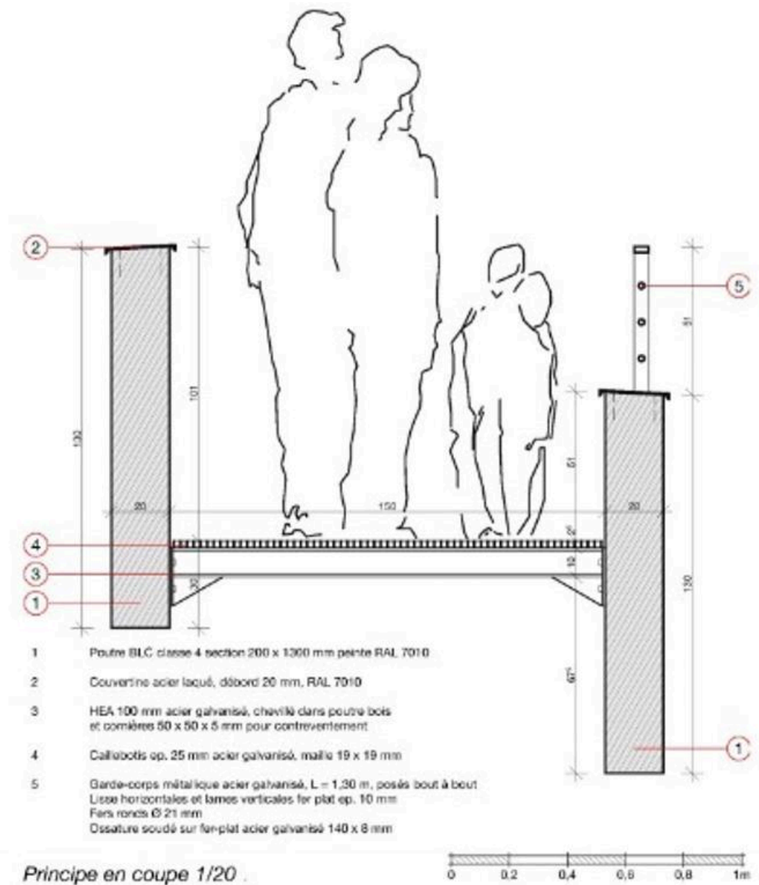
Passerelle de l'Abbaye d'Aulps, principe en coupe
