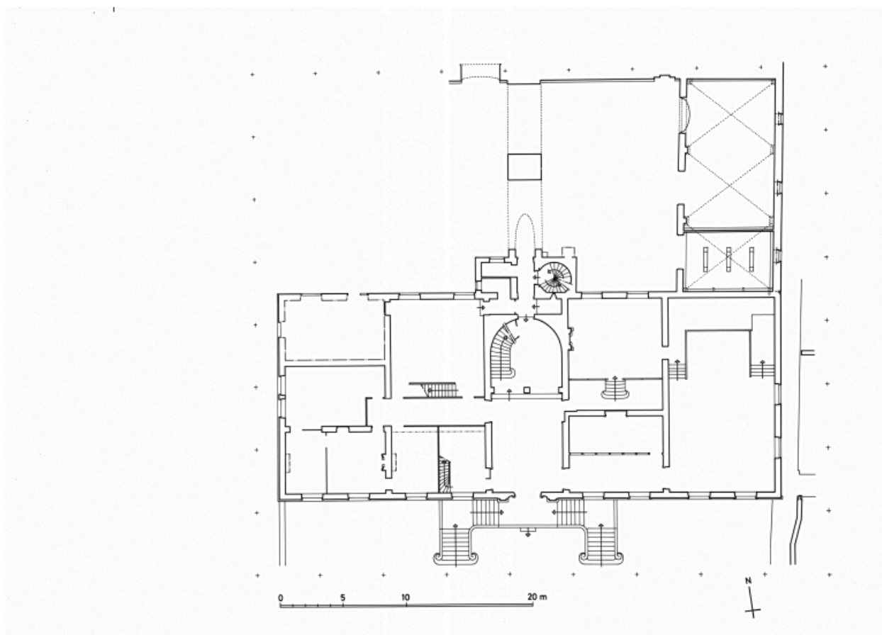
Plan du rez-de-chaussée surélevé, relevé expédié et schématique. Rel. Inv. P. Cherblanc, 1991
