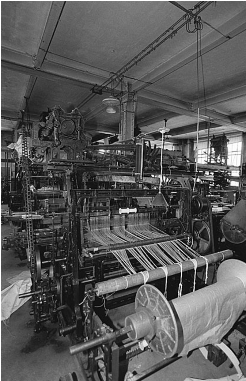
Métier n° 20 à mécanique ratière, vue nord-est
