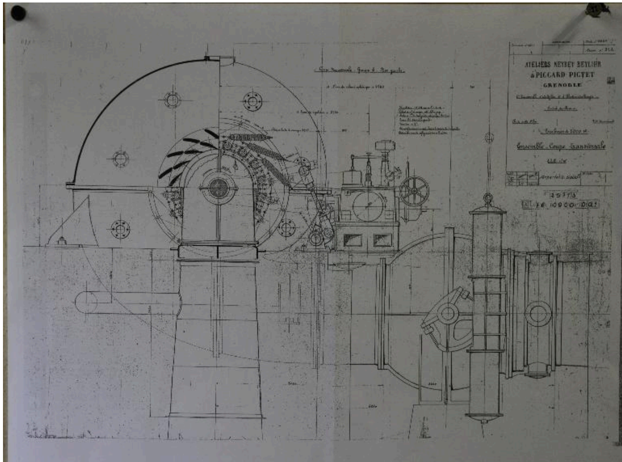
Coupe tra,seversale d'origine d'une bobine produite par les ateliers de Neyret-Bellier & Piccard-Pictet à Grenoble
