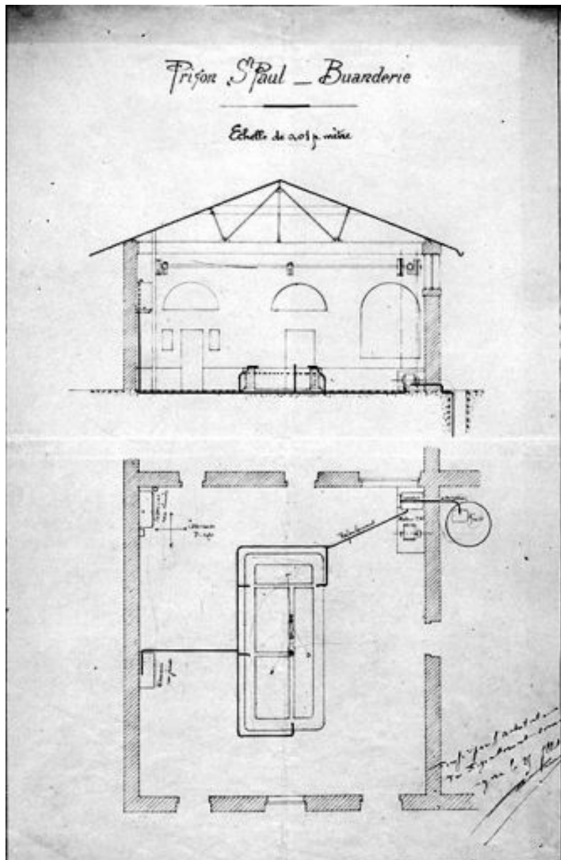
Coupe et plan de la buanderie avec installation d'une pompe, 1901
